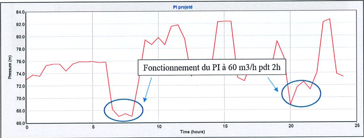
Figure 3 : Résultat modélisation numérique du PI projeté
